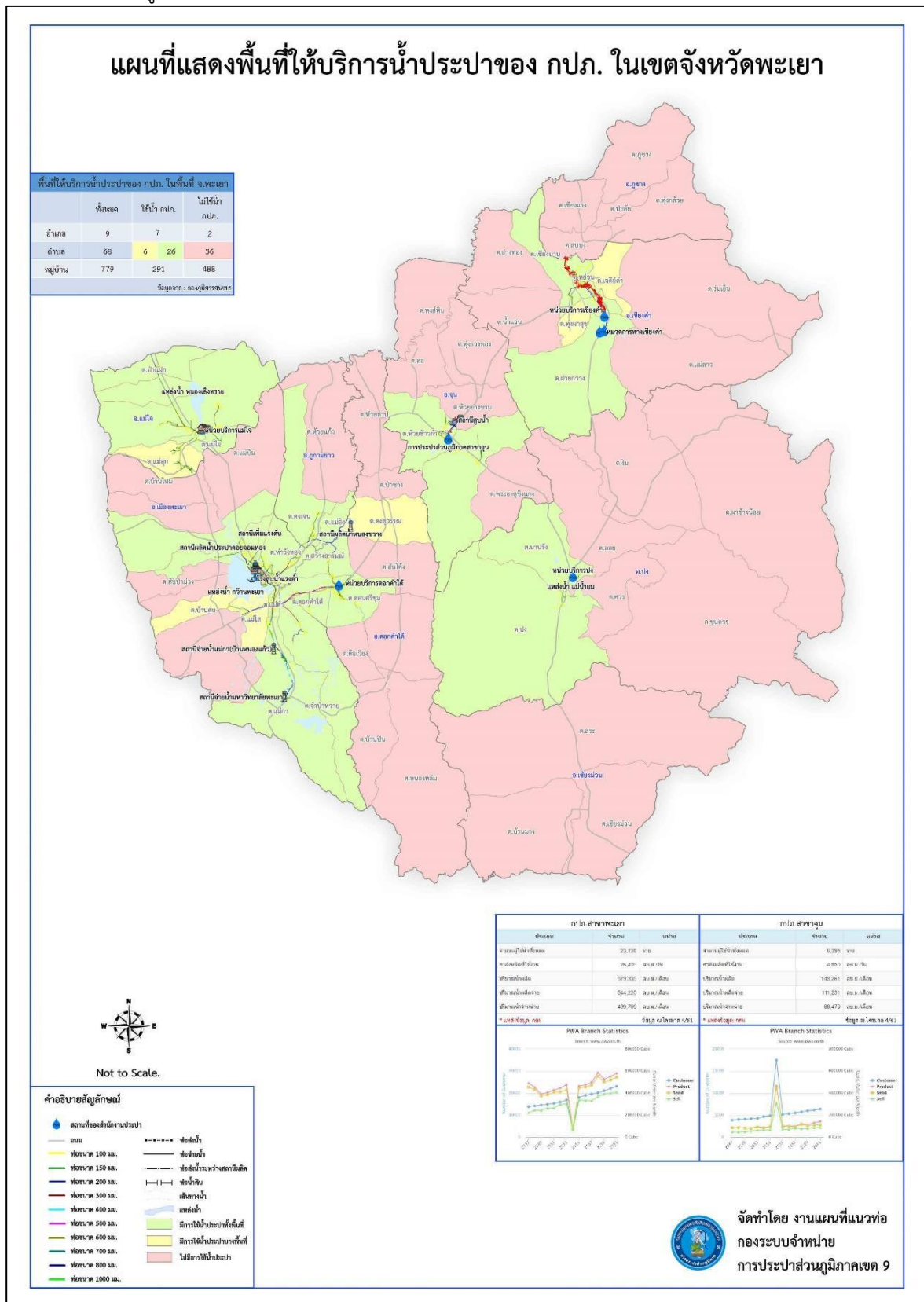
รูปที่ ๑๐ แผนที่แสดงพื้นที่ให้บริการน้ำประปาของ กปภ. ในเขตจังหวัดพะเยา
